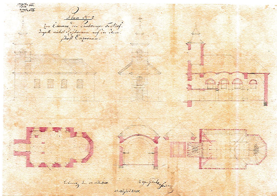
Obr. 6. Plán novostavby kaple sv. Václava od Wenzela Gerzabka z 28. 2. 1830 se změnami zakreslenými 28. 8. 1831, SOA Litoměřice, Vs Encovany.
